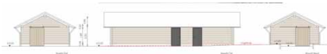
Ansicht Süd
